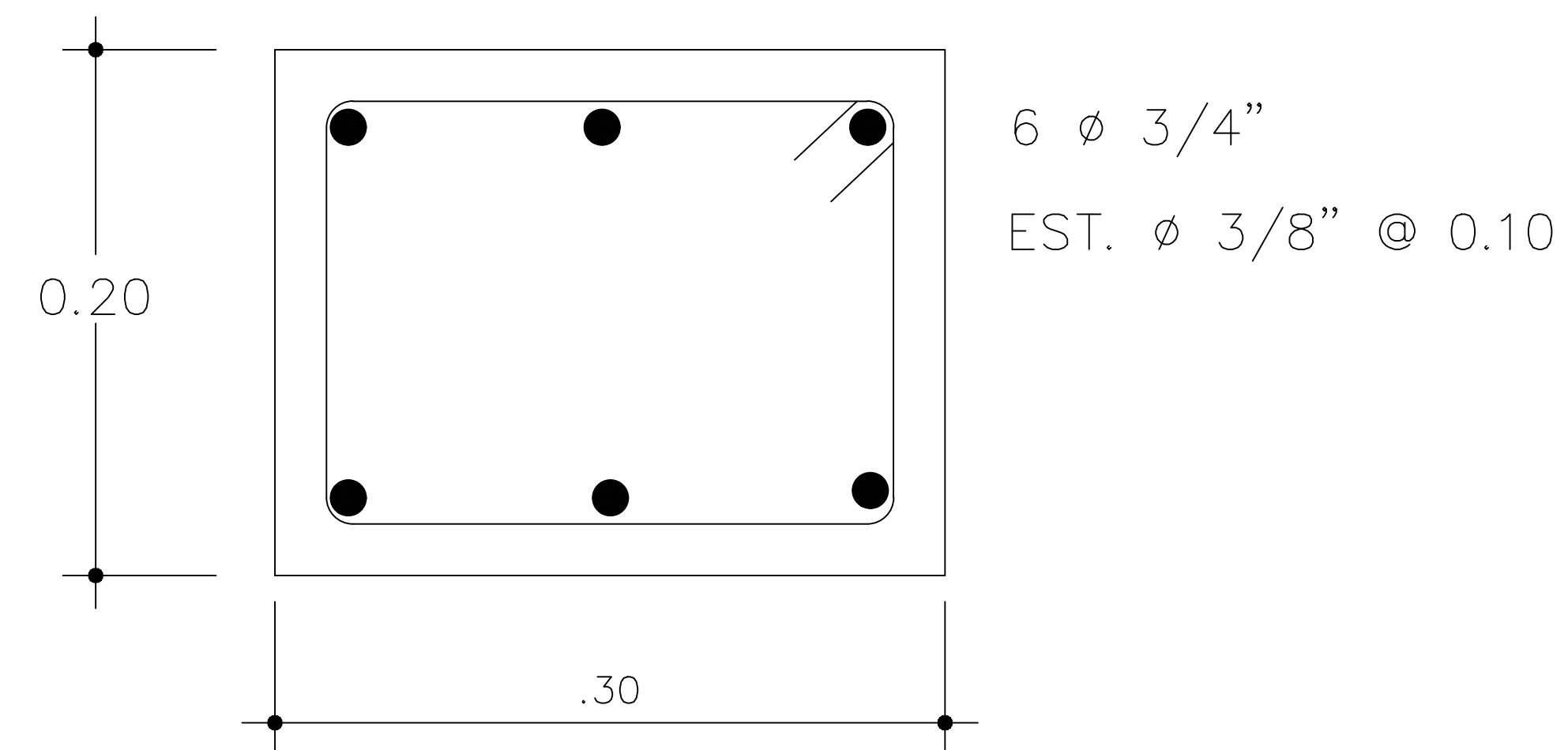
SECCION 3-3' : seccion transversal viga
