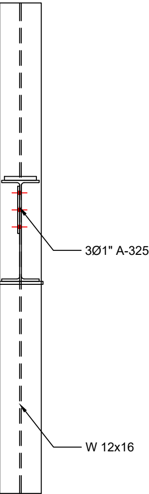
Detalle conexion viga - columna D-2
