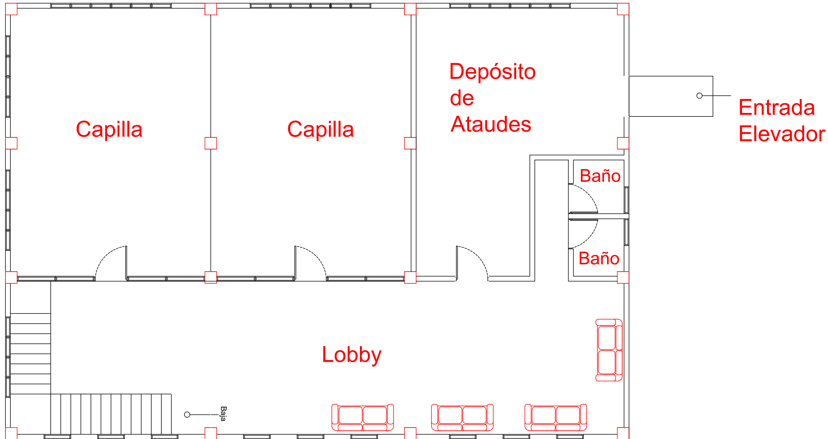
Planta Amueblada 2do Nivel
