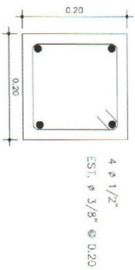
Detalle de columna
