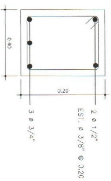
Detalle de viga de carga
