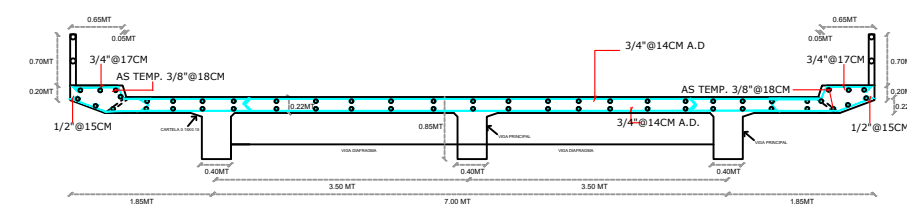
SECCIÓN C-C'
