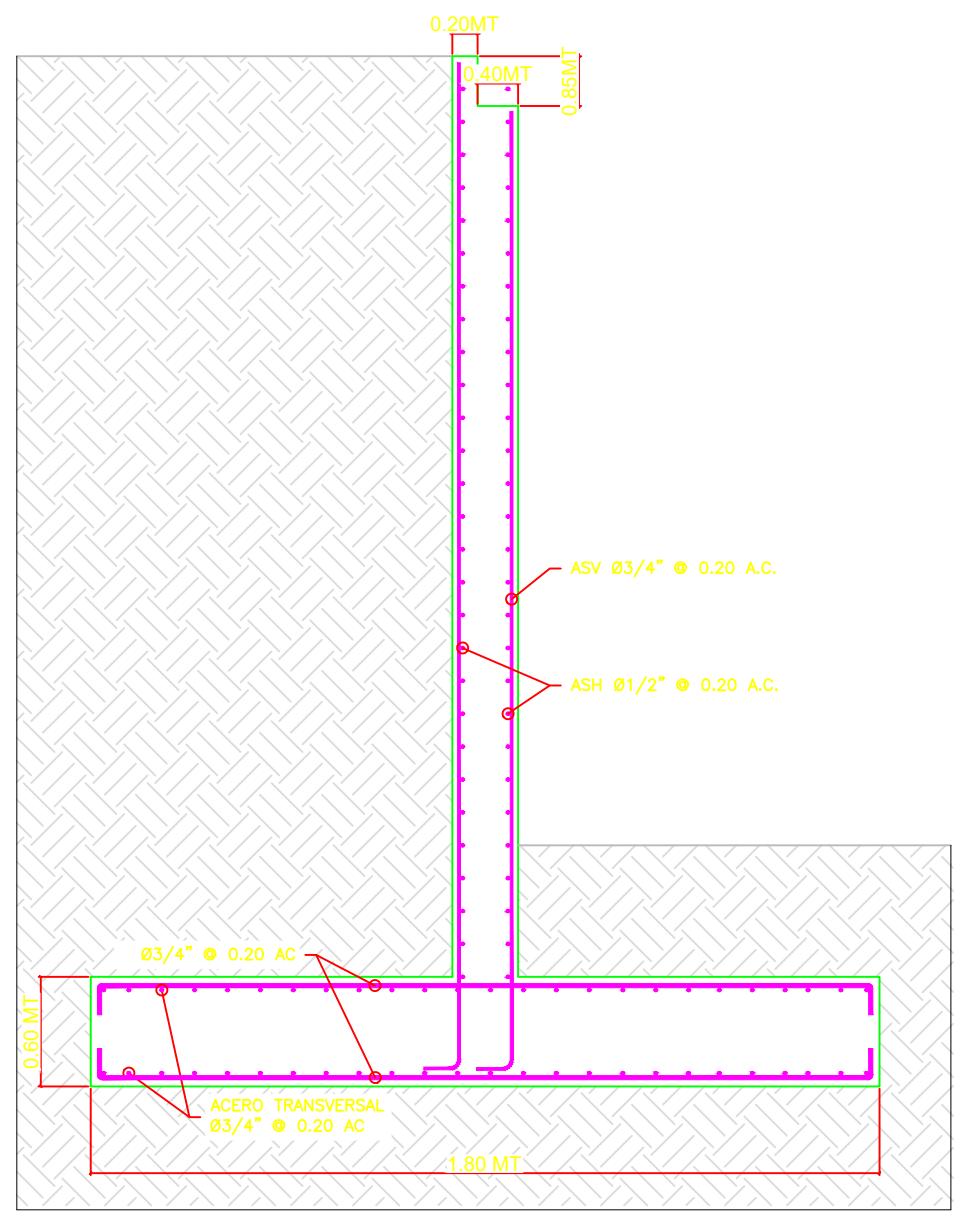
SECCIÓN A-A'
