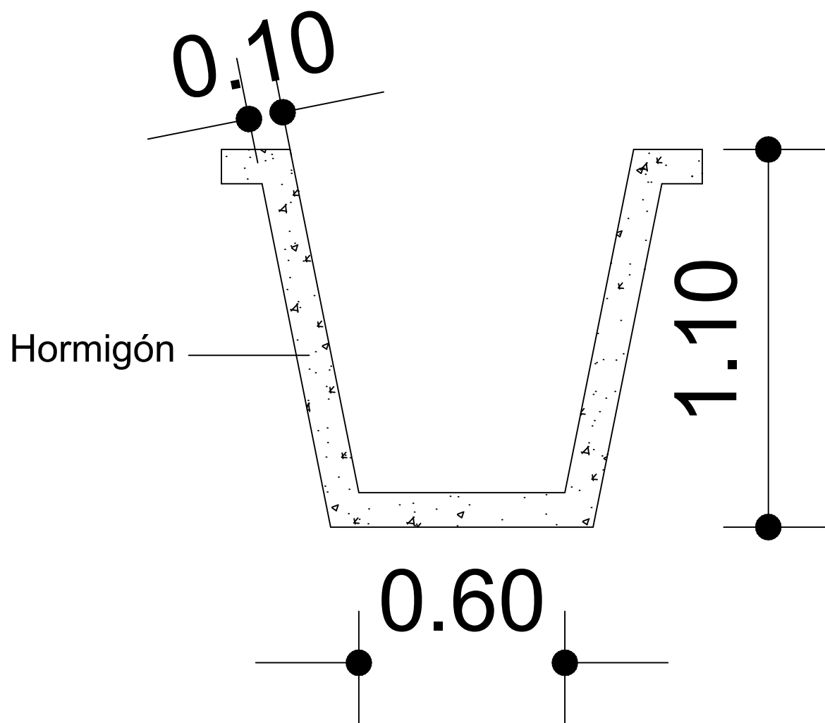
Detalle Canaleta
